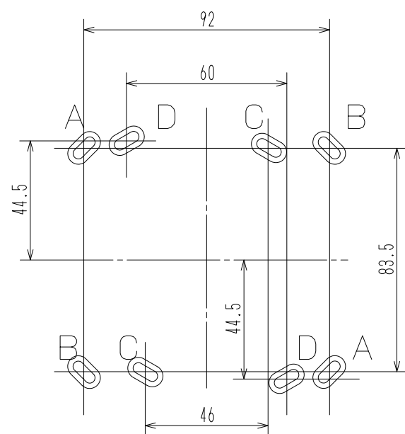
取付穴寸法図 S=1/2
