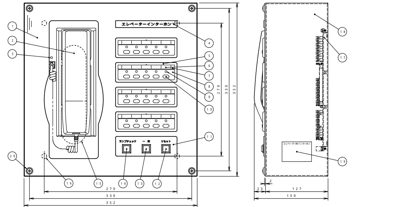
外形図 (EZS - 05K・10K・15K・20K)
