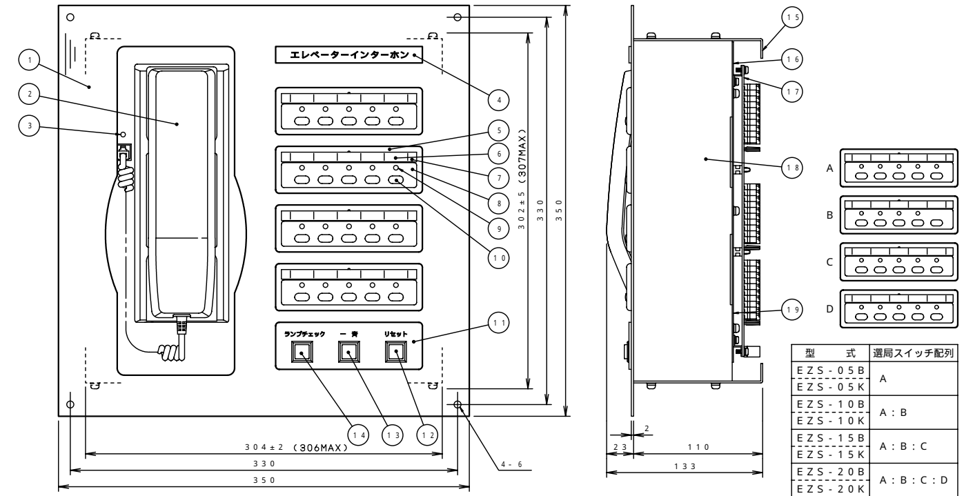
外形図 (EZS - 05B・10B・15B・20B)
